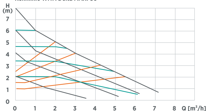
Kennlinie WITA Delta MAXI 80
