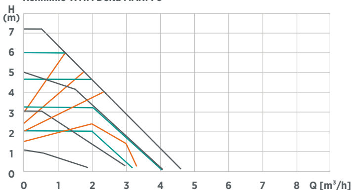
Kennlinie WITA Delta MAXI 70
