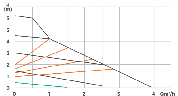
Kennlinie WITA Delta TOP 60
