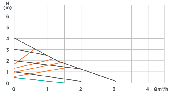
Kennlinie WITA Delta TOP 40
