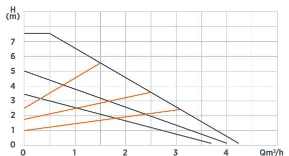
Kennlinie WITA Delta Plus UE 75A
