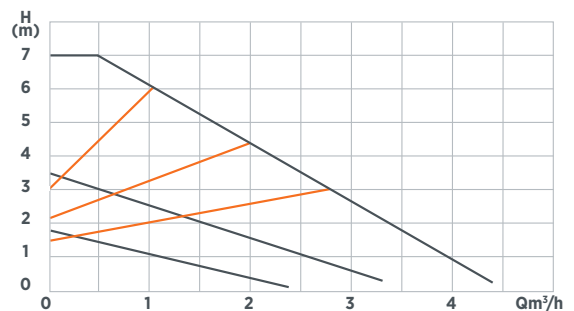
Kennlinie WITA Delta Plus UE 70A
