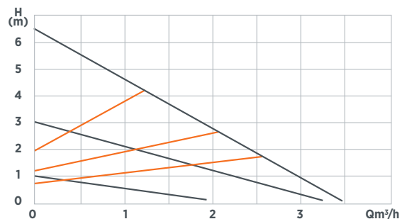
Kennlinie WITA Delta Plus UE 55A
