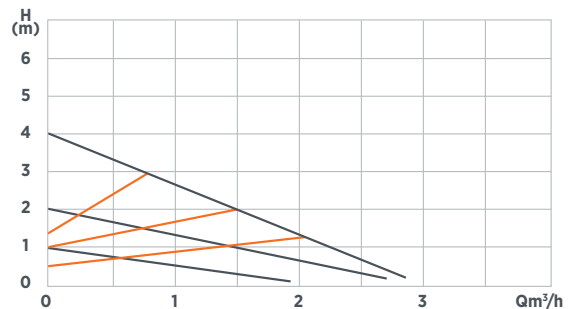
Kennlinie WITA Delta Plus UE 35A
